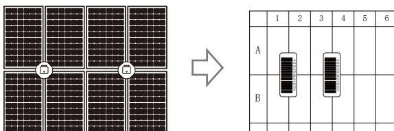
Abbildung Die Installationskarte (TSOL-M1600)
