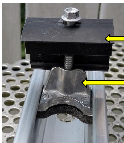
Abb. 14/ vormontierte Modulklemme
