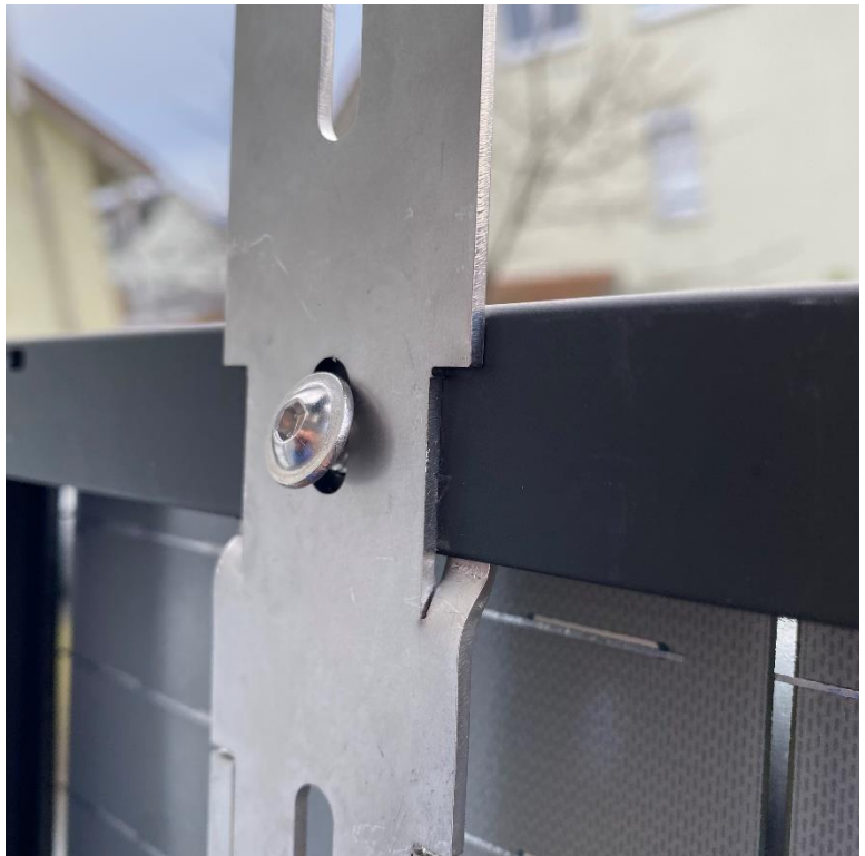
Abb. 5/locker angesetzte Schraube M6 kurz
